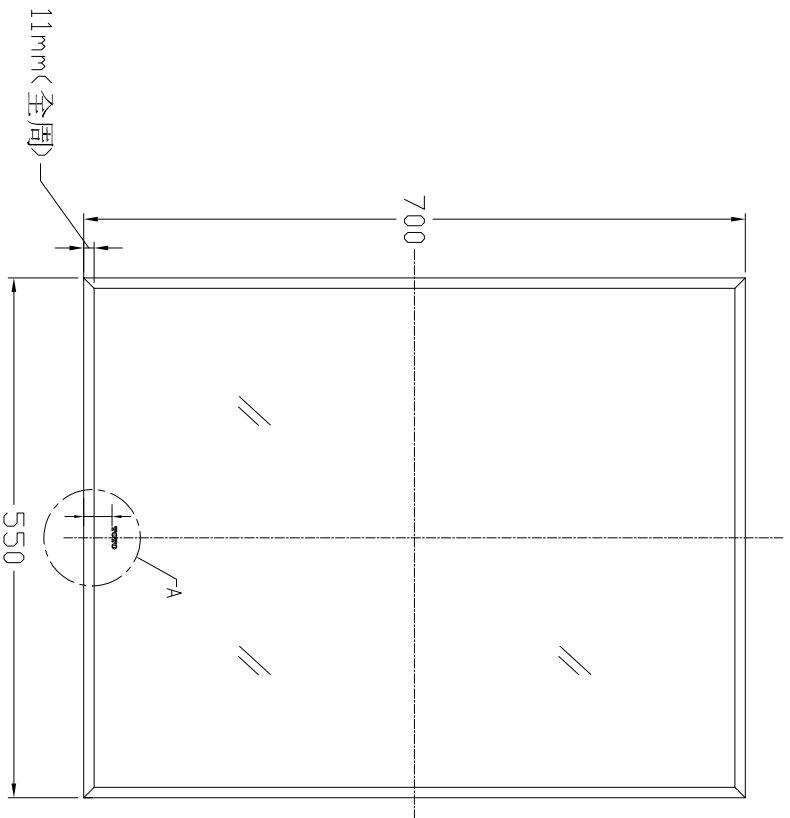
正視圖
